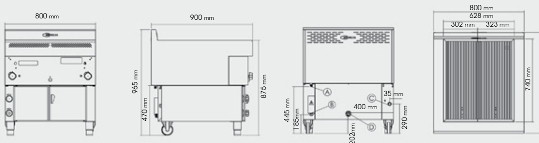
GHPI 2/800
